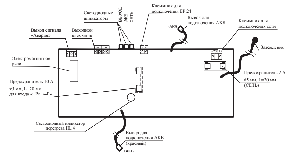
Рисунок 1– Плата источника
